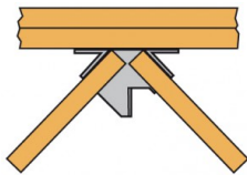
2 arêtiers sans empannon
