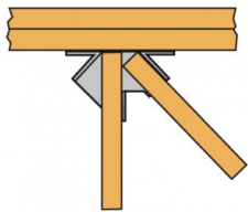
1 arêtier + 1 empannon
