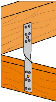
Bevestiging van 2 loodrechte kepers met SUT
