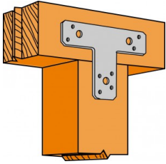
T-bevestiging met 66T
