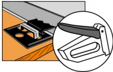
Bevestiging van de WPC met nieten
